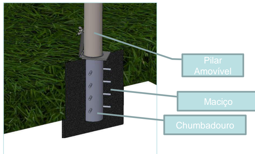
Chumbadouro do Pilar amovível com tampa de proteção
